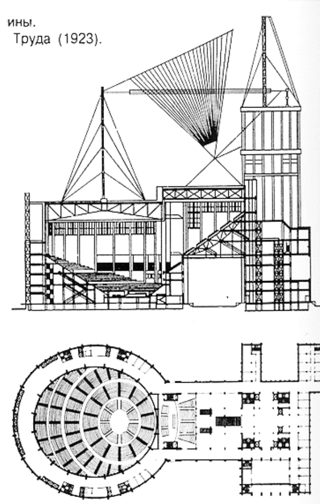
ヴェスニン兄弟設計による 労働宮殿コンペ案 1922-23年
